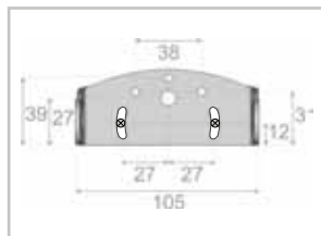
ブラケット寸法
